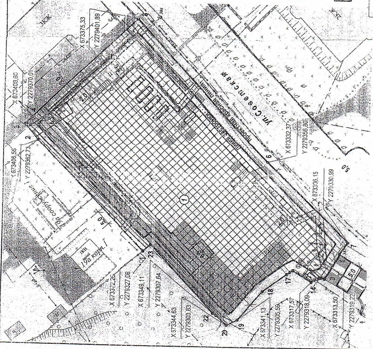
1. Чертеж градостроительного плана земельного участка
