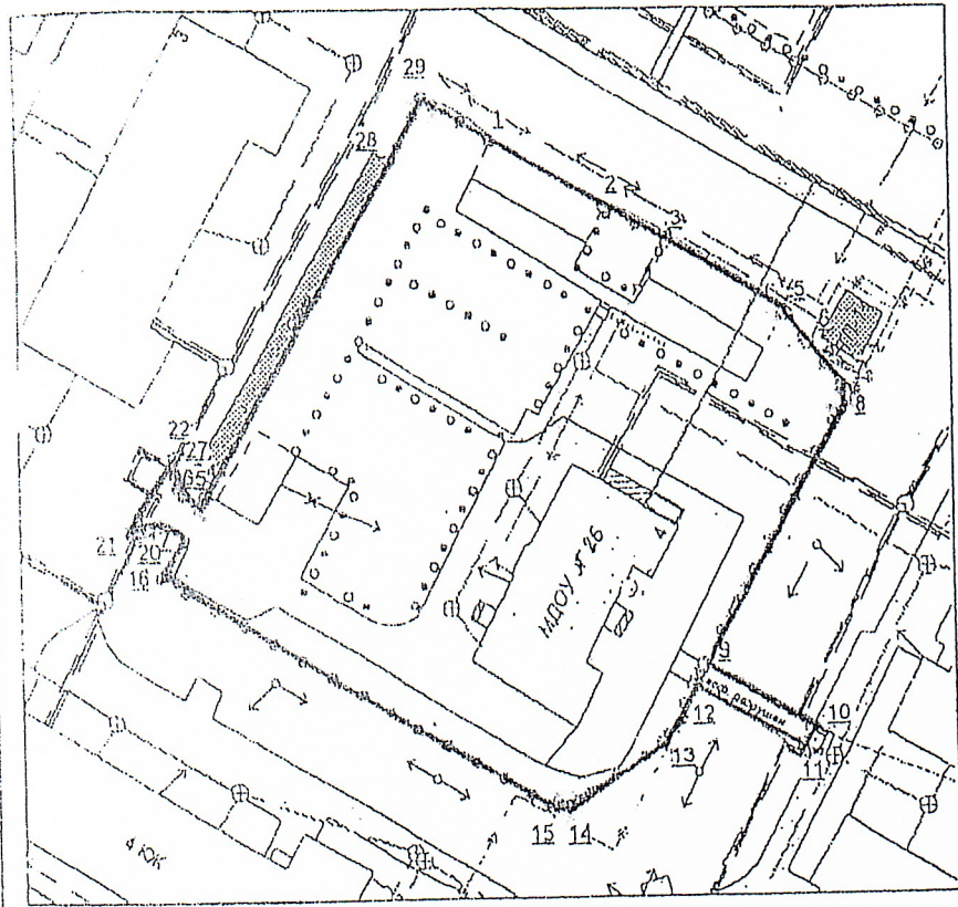
Масштаб 1: 1000
