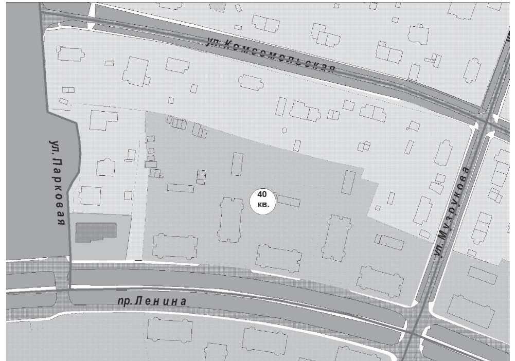
Графическое изображение фрагмента Схемы генерального плана (основной чертеж) Генерального плана города Озерска (инв. № 308-211ДСП, лист 6) (кадастровый квартал 74:41:0101021)
